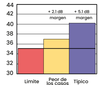
Pérdida de FEXT a 250 MHz (dB)
