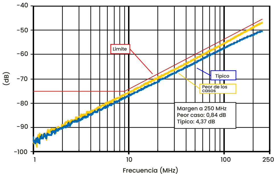
Rendimiento de diafonía en el extremo cercano
