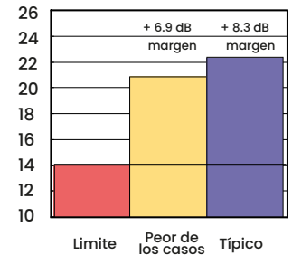
Pérdida de retorno a 250 MHz (dB)
