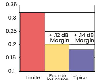
Atenuación a 250 MHz (dB)
